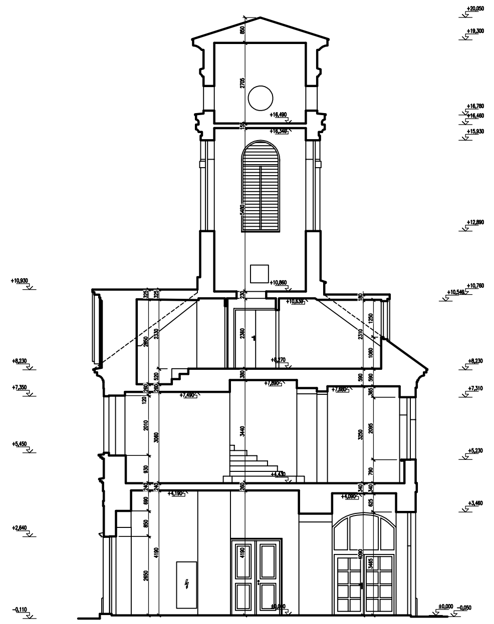
REZ B-B
