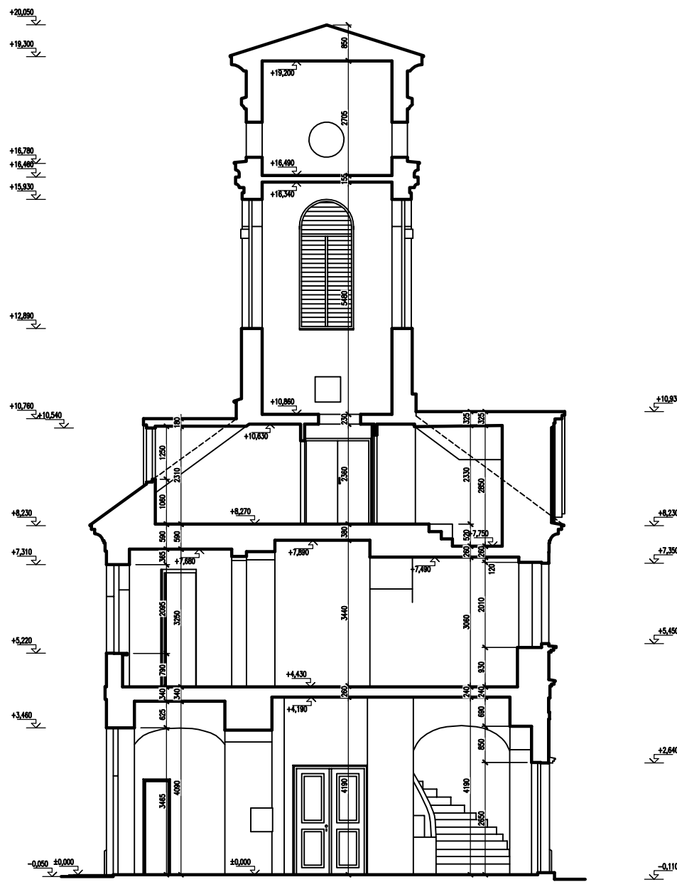
REZ A-A
