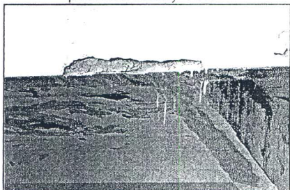
poškodená omietka podhľadu terasy
